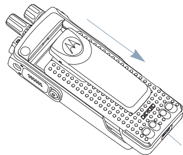
Фиксатор аккумулятора
